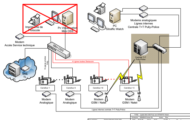
Schéma du nouveau système de régulation (source: Siemens)
